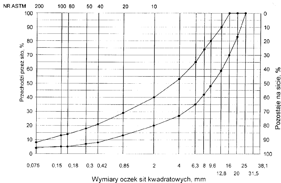
Rys. 1. Krzywe graniczne uziarnienia mieszanek mineralnej BA od 0 do 20 mm do podbudowy nawierzchni drogi o obciążeniu ruchem KR 2
