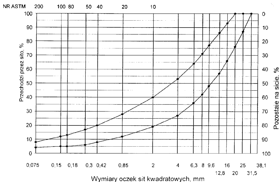
Rys. 1. Krzywe graniczne uziarnienia mieszanki mineralnej BA od 0 do 25mm do podbudowy nawierzchni drogi o obciążeniu ruchem KR 2
