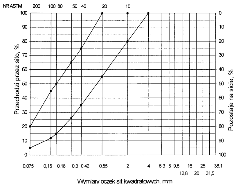
Rys.1. Krzywe graniczne mieszanki mineralnej asfaltu piaskowego
