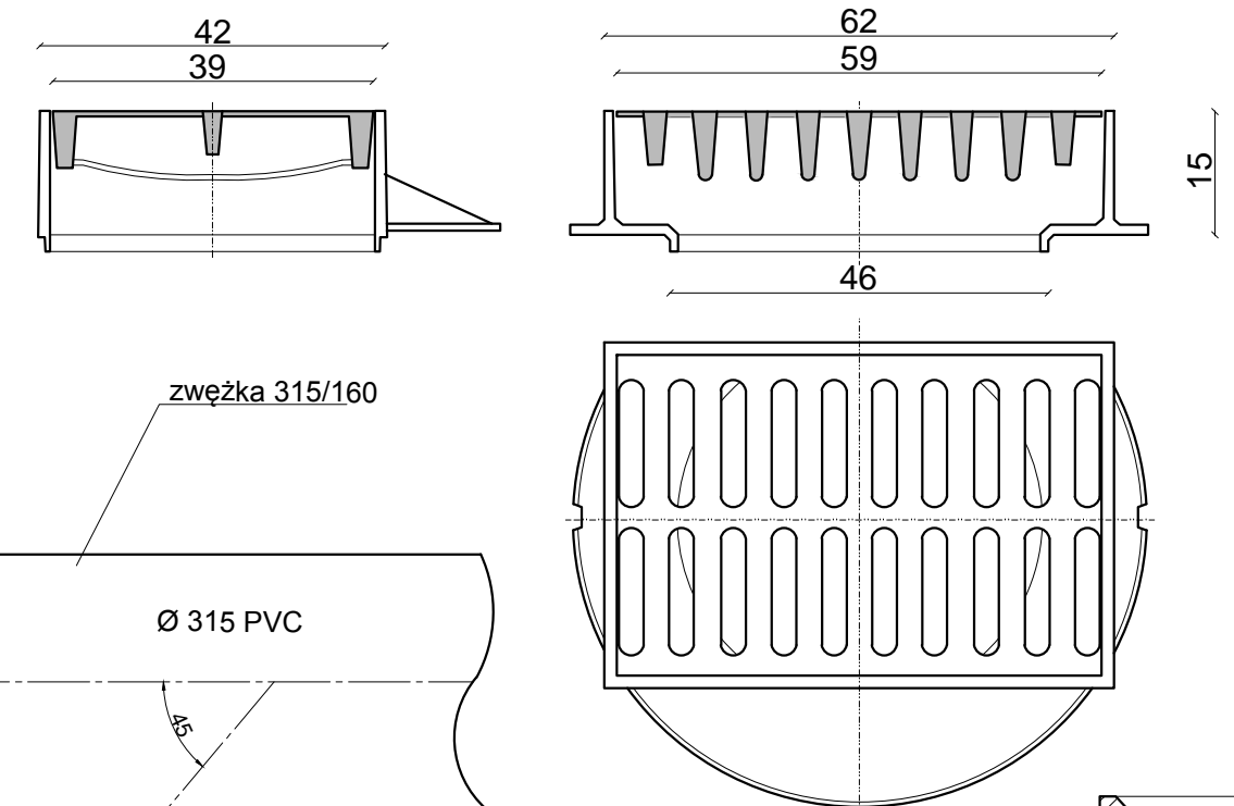
Widok A-A
