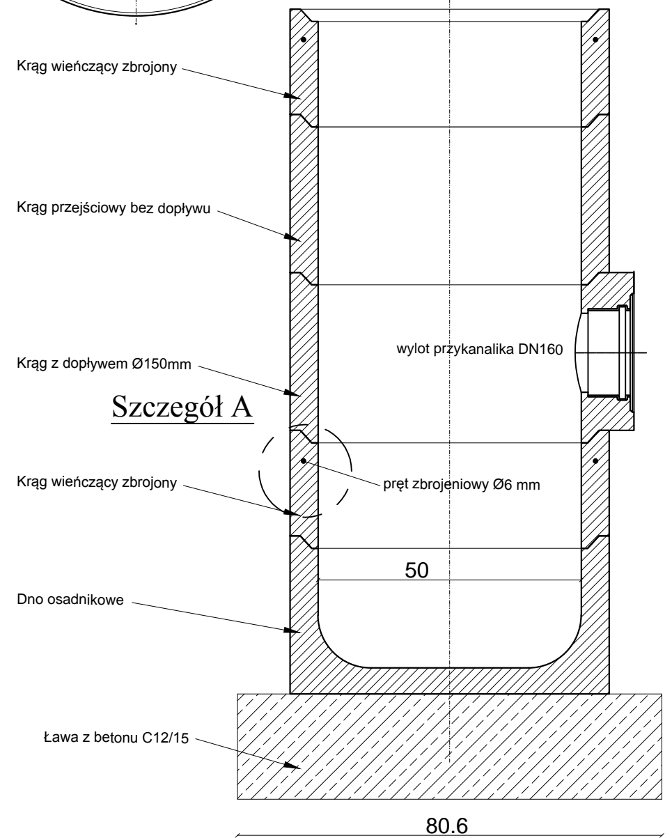
Widok A-A
