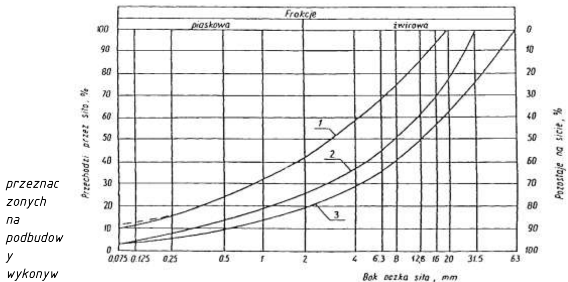
Rysunek 1. Pole dobrego uziarnienia kruszyw
