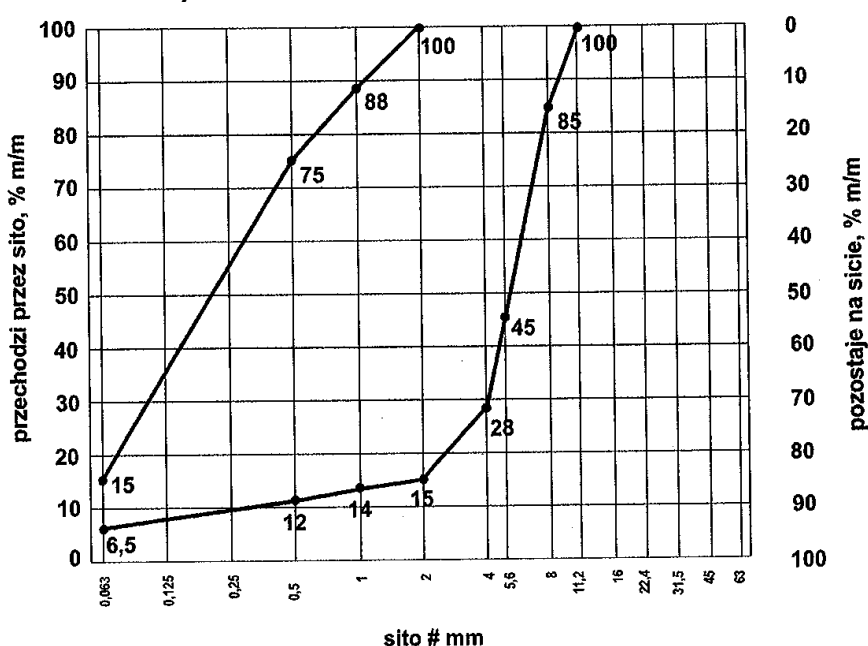
Rys. .1.2 Uziarnienie mieszanki CBGM 0/8
